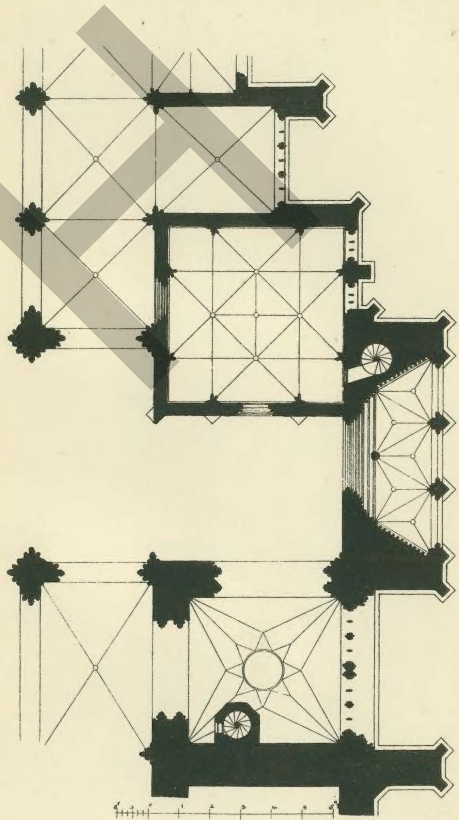
Jindřys jižní křížové lode, věže a kaple Svatováclavské. Starý škov.
